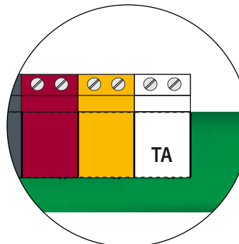
Płytki zaciskowe Bus modułu
